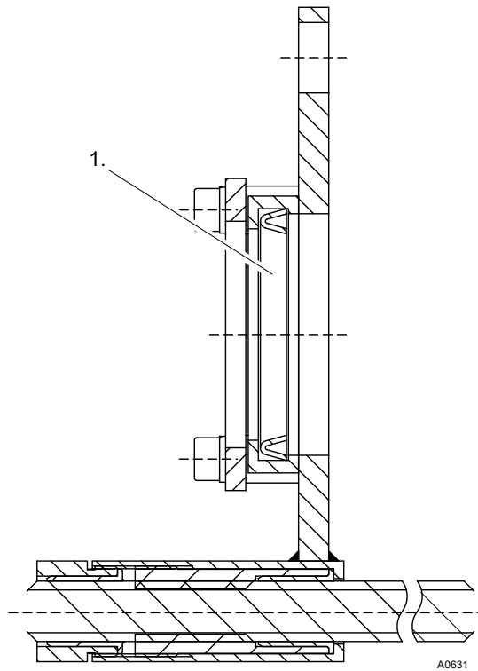
Fig. 37: Wiper element
