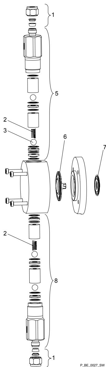
Fig. 15: Beta® 0708 (1008) - 0220 (0420) SS liquid end
