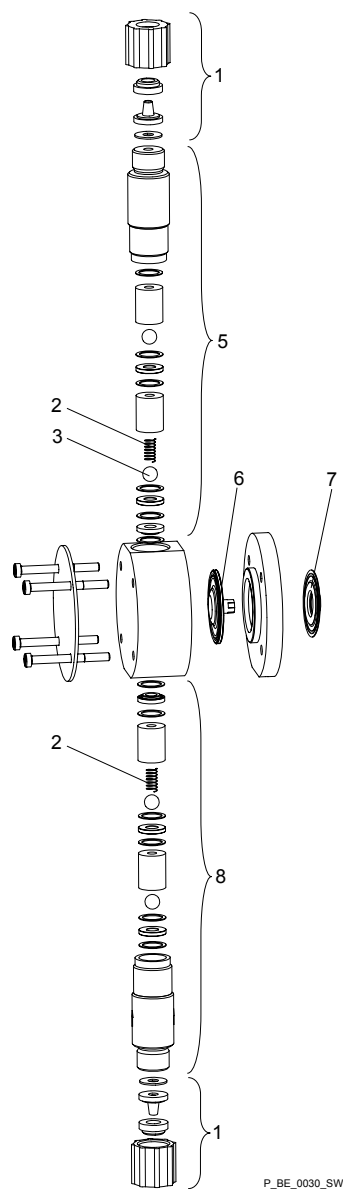
Fig. 12: Beta® 0708 (1008) - 0220 (0420) TT liquid end
