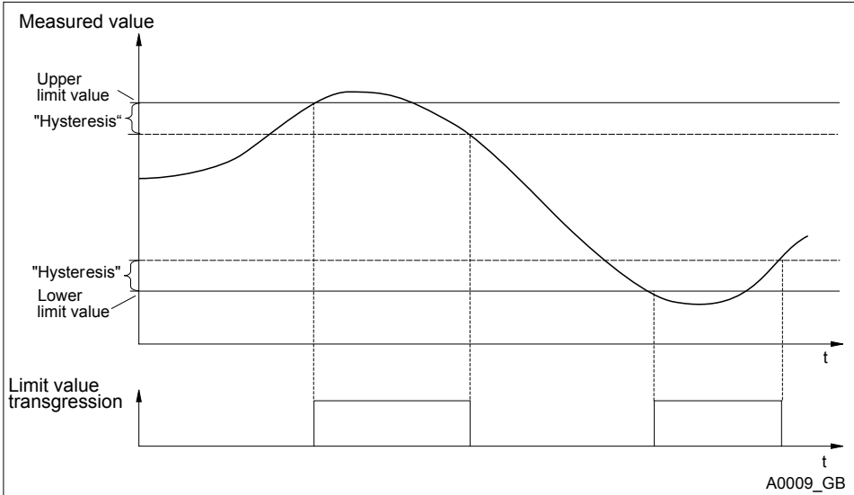
Fig. 80: Hysteresis
