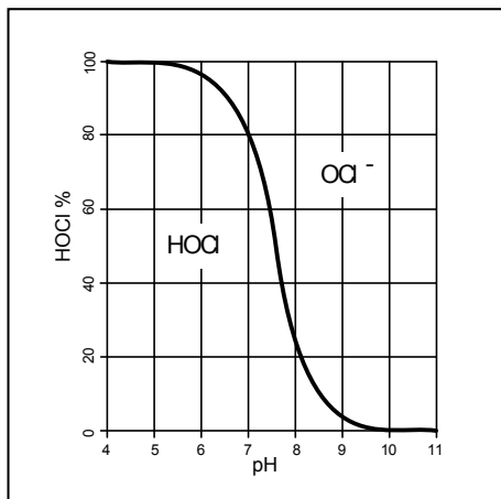
Fig. 32: HOCl/OCl - equilibrium
