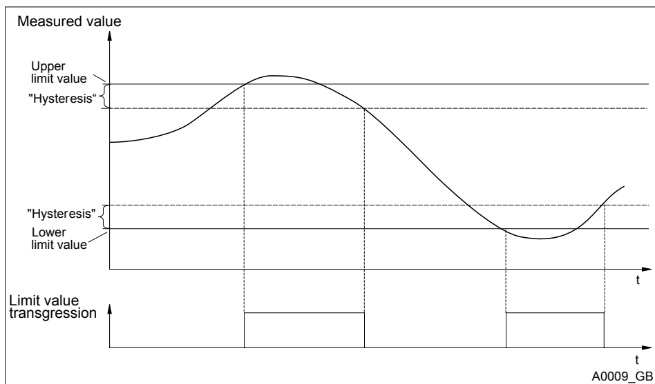
Fig. 35: Hysteresis
