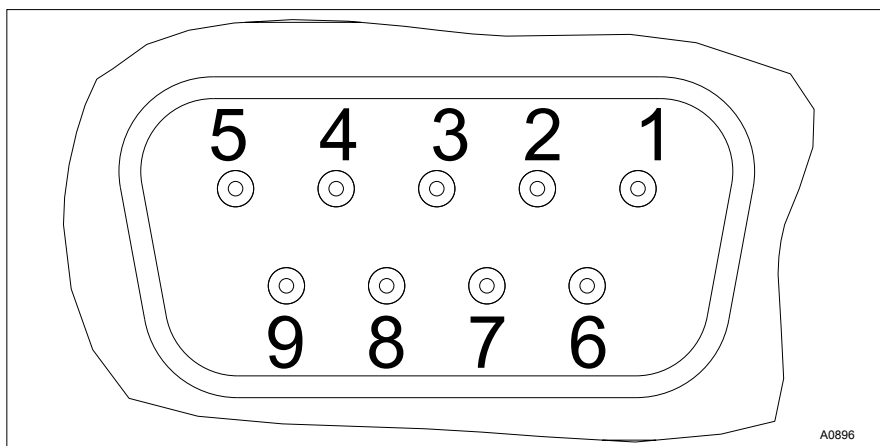
Fig. 4: D-sub socket
