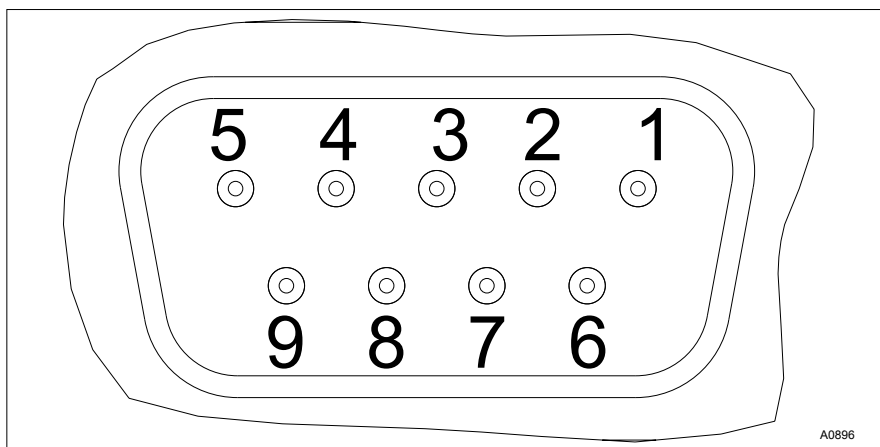
Abb. 4: D-Sub-Buchse
