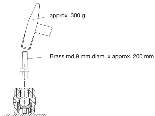
Fig. 18 S3Ba/S3Ca-019-GB
