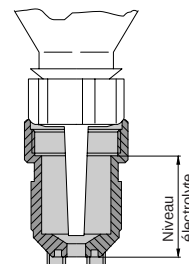
Fig. 2 : Capuchon de membrane
