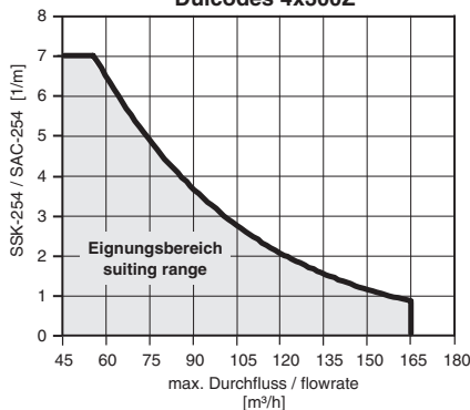
Auslegungsdiagramm / design diagram Dulcodes 4x300Z
