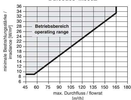
Betriebsdiagramm / operating diagram Dulcodes 4x300Z
