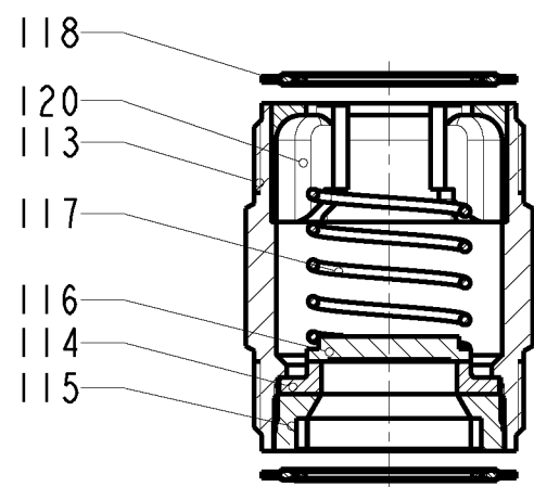
Pos. 101 Ventil kpl. Hast.C Valve cpl. Hast.C
