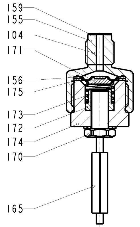
Pos. 104 Membr.Bruchmelder kpl. 2m NAMUR SST Diaphr.br.signal cpl. 2m NAMUR SST
