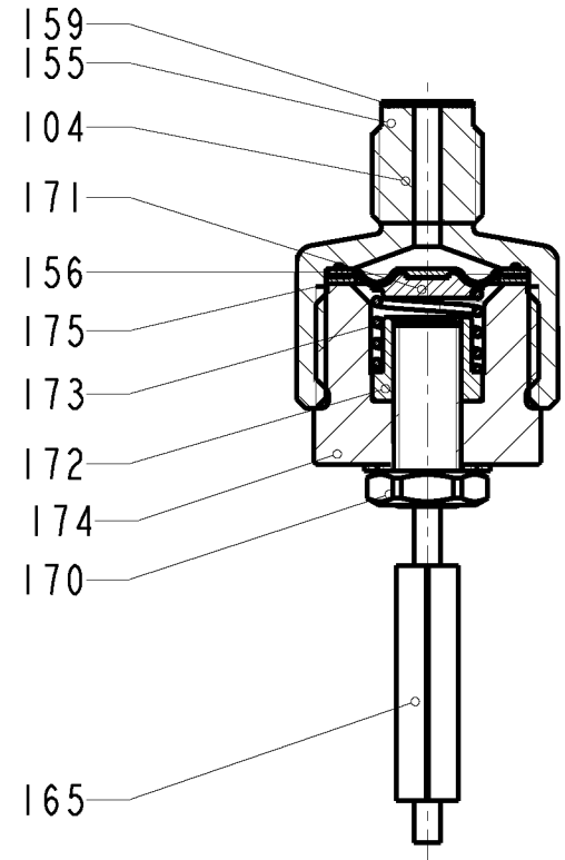
Pos. 104 Membr.Bruchmelder kpl. 2m NAMUR SST Diaphr.br.signal cpl. 2m NAMUR SST
