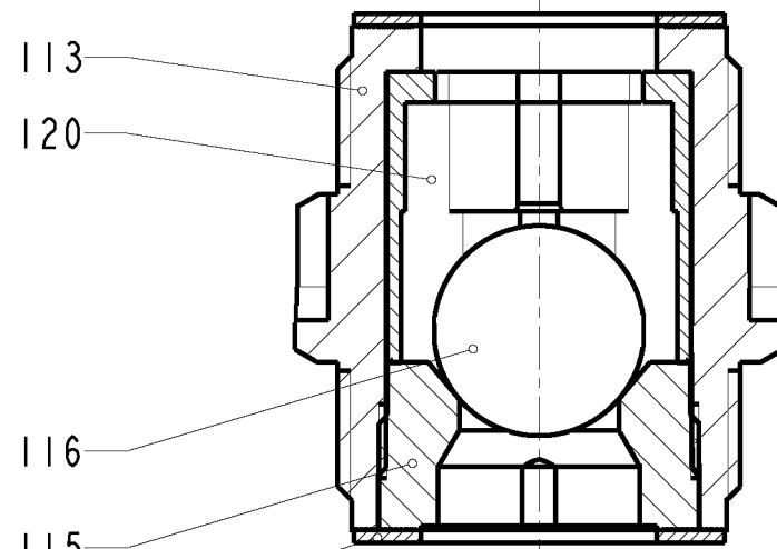
Pos. 101 Ausführung HCT Ventil kpl. Hast.C Design HCT Valve cpl. Hast.C
