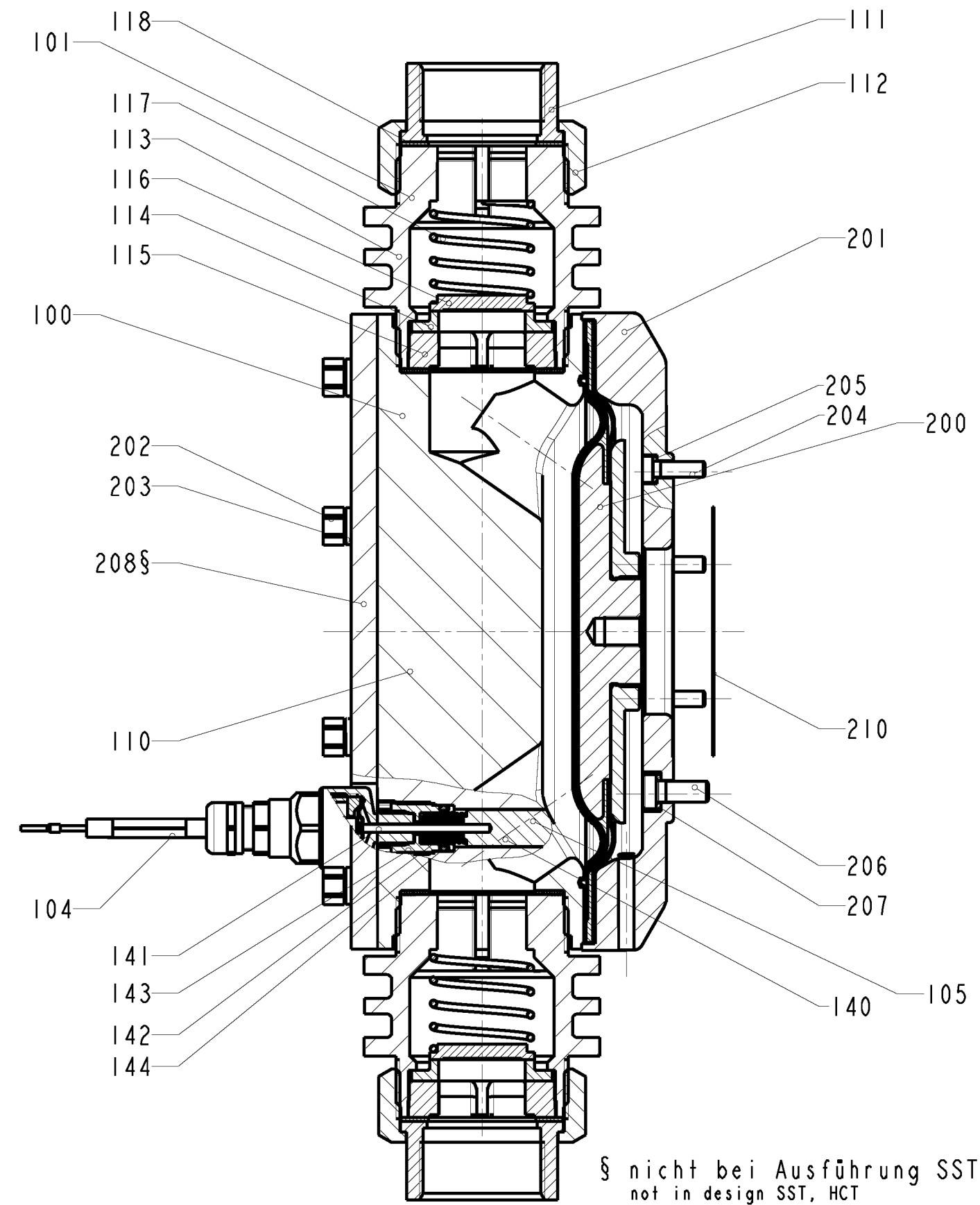
Pos. 104 Membr.Bruchmelder kpl. 2m NAMUR SST Diaphr.br.signal cpl. 2m NAMUR SST
