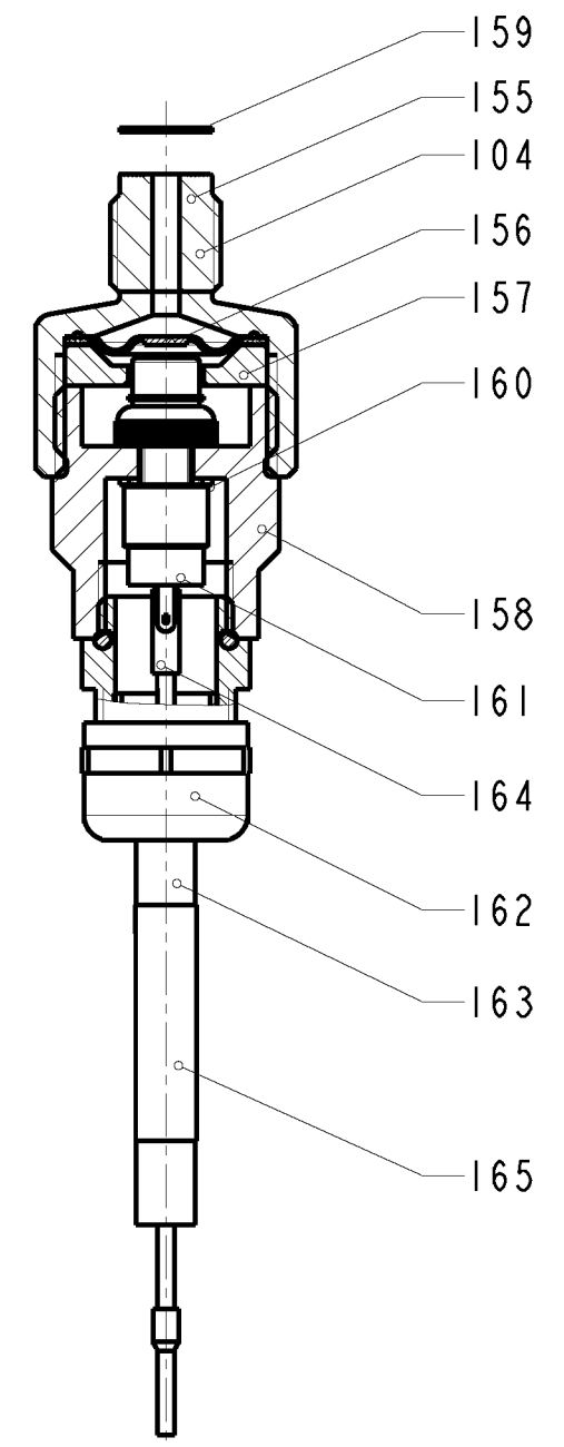
Pos. 104 Membr.Bruchmelder kpl. 2m KONTAKT SST Diaphr.br.signal cpl. 2m CONTACT SST
